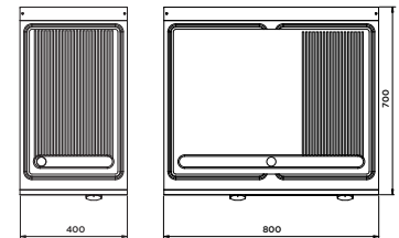
PLAQUE LISSE/NERVURÉE ACIER INOXYDABLE BRATPLATTE GLATT/GERILLT ROSTFREIER STAHL
